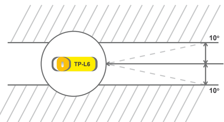
Rys.: Sposób wyznaczenia spadku (rys. górny) i kierunku (rys. dolny) za pomocą lasera liniowego wstawionego do studzienki kanalizacyjnej
